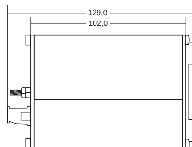
LATERAL dimensiones en mm
